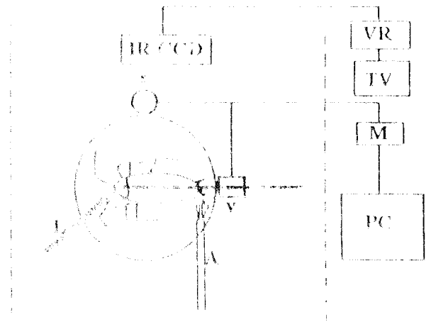
圖 1 實驗裝置。本設計用於偵測蟑螂在圓球上生活與逃自行爲。實驗用蟑螂在木架固定足跡在保麗龍球上，並利用鼠為記錄外在刺激因子的實驗裝置。X、Y 的兩個方向偵測昆蟲逃自行爲，X 為垂直方向，Y 為水平方向。A：空氣刺激，IR-CCD：紅外線攝影裝置，L：光刺激，M：滑鼠系統，PC：個人電腦，TV：電視機，VR：錄影機。
