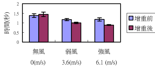
圖四 種子增重後之飄落時間比較圖 (n=48)
