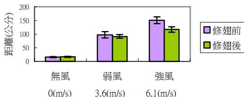
圖九 種子寬翅修剪前後飄散距離之比較圖 (n=46)
