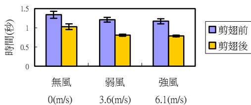
圖六 種子剪翅前後的飛行時間比較圖 (n=48)
