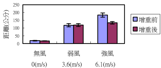
圖五 種子增重後之飄散距離比較圖 (n=48)
