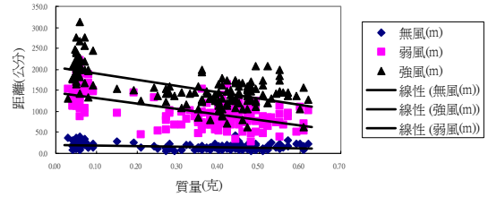
圖三 種子質量與飛行距離關係圖(1.5m 高)
