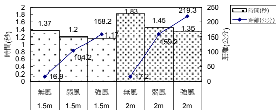
圖十 桃花心木種子飛落時的高度與飄落時間及飄散距離之關係圖
