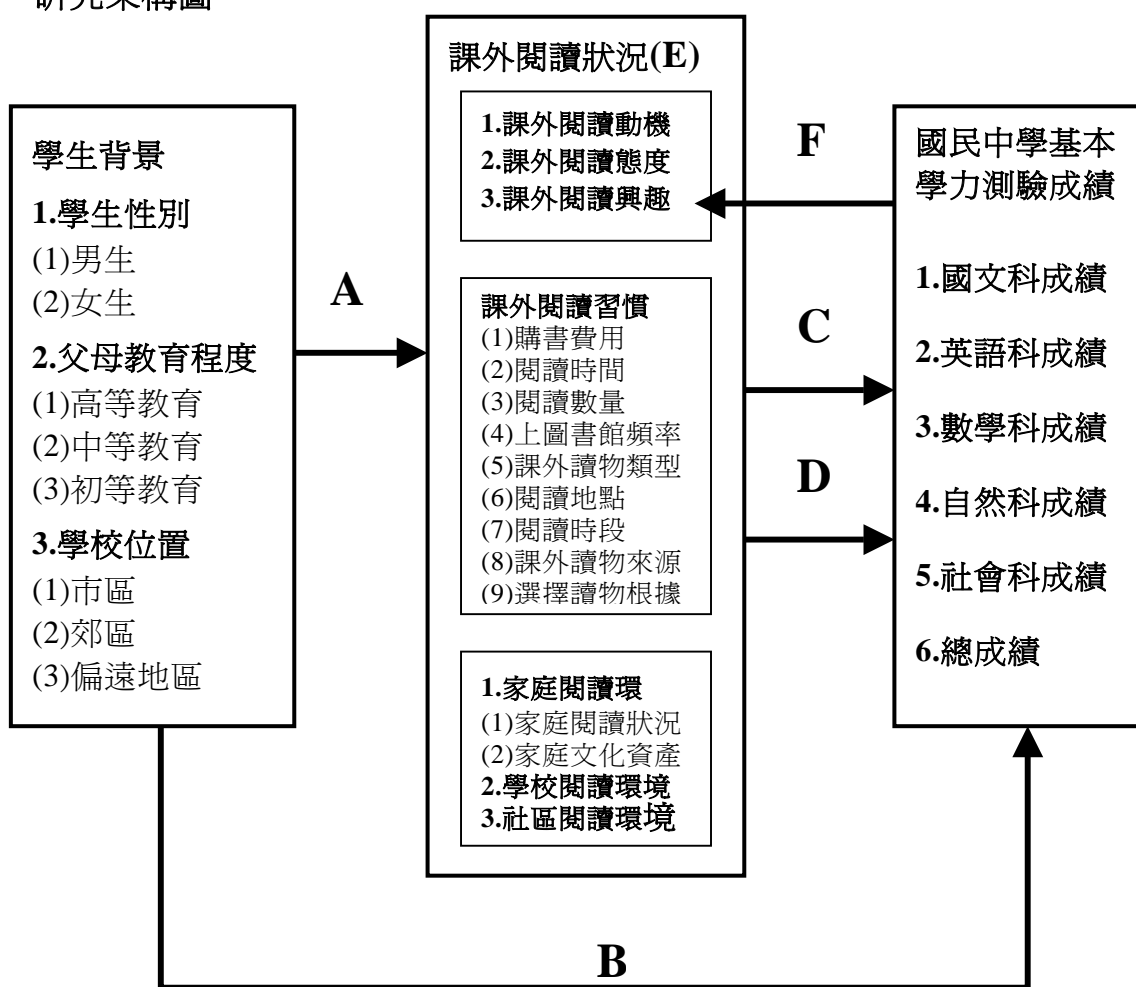
圖 3-1-1 研究架構圖
